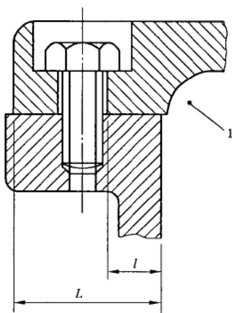
图 3 平面接合面上的孔(一)
