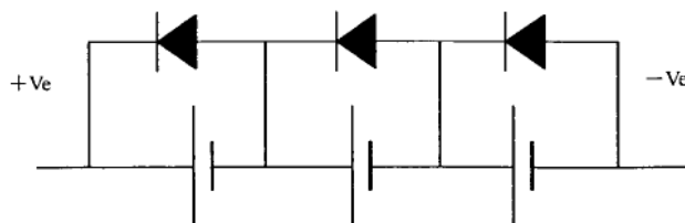
图 E.1 为三个串联单体电池安装的二极管
