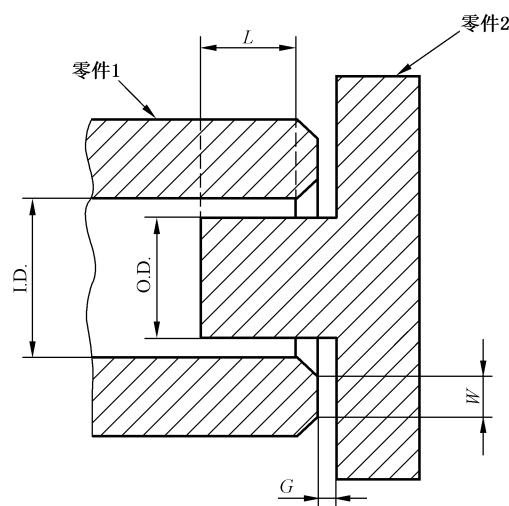
图 2 止口接合面
