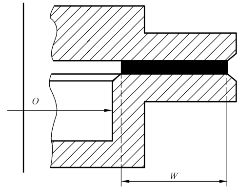
图 3 衬垫接合面
