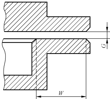
图 1 平面接合面
