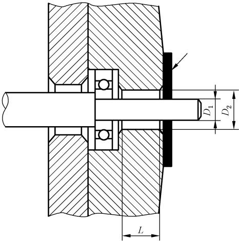
图 4 转速等于或大于 100 r/min 的转轴
