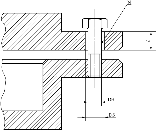
图 5 螺杆间隙
